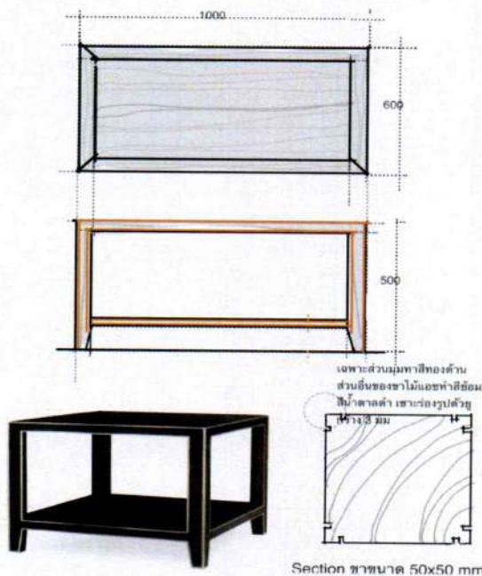
ภาพแสดงรายละเอียดส่วนตัวทองปลิง 6 มม. ทาสีทองด้าน
