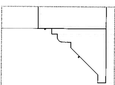
DETAIL-A SCM 1:2
